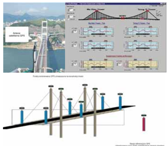
Rys. 3. Przykład instalacji systemu monitoringu konstrukcji mostu – schemat rozmieszczenia punktów wraz z przykładem analiz prowadzonych w czasie rzeczywistym; źródło: Leica Geosystems AG
