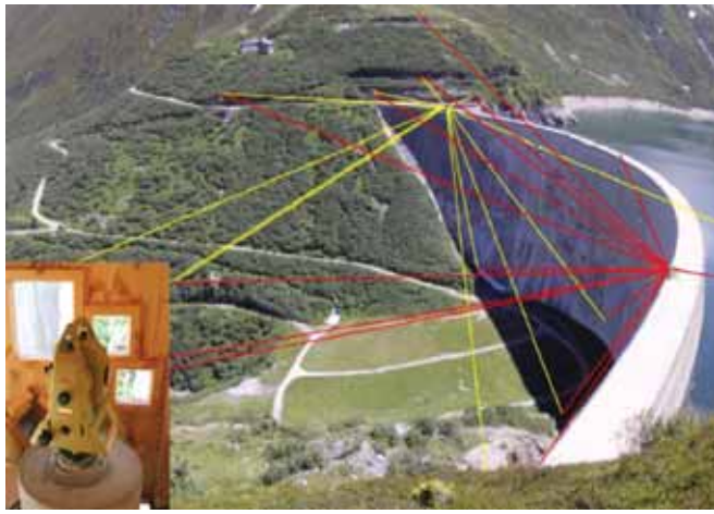
Rys. 4 Przykład instalacji dynamicznego systemu monitoringu zapory wodnej (stałe stanowisko tachymetryczne wykonujące ciągły pomiar sieci kątowno-liniowej); źródło: Leica Geosystems AG
