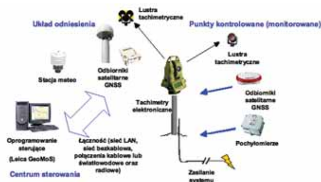
Rys. 1. Ogólny schemat budowy systemu monitoringu inżynierskiego na przykładzie Leica GeoMoS
