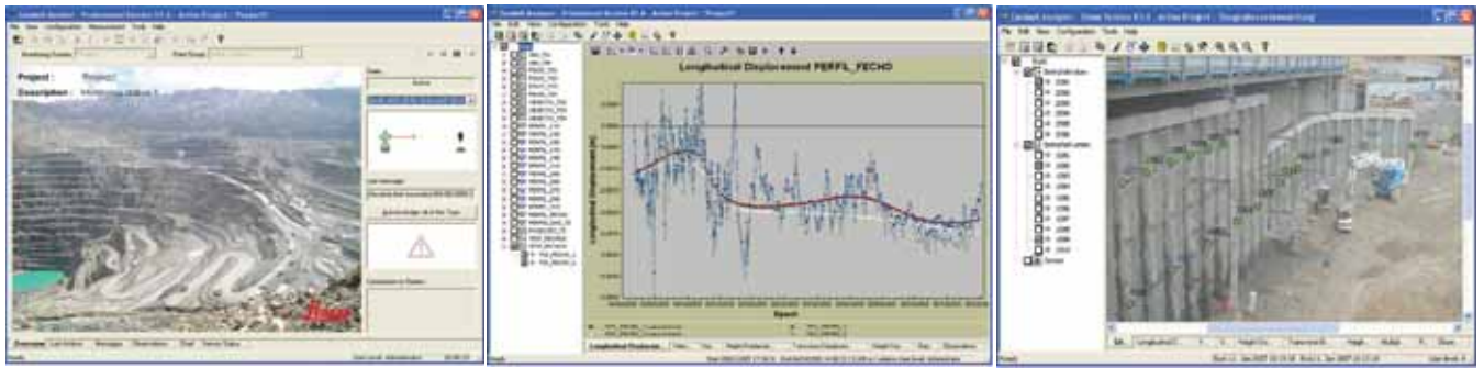
Rys. 2. Widok okien dialogowych modułów aplikacji Geodetic Monitoring System – GeoMoS
